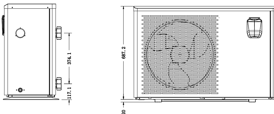
Värmepump 1402, 1403 och 1404
