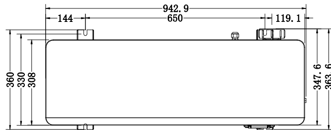
Lämpöpumppu 1402, 1403 ja 1404
