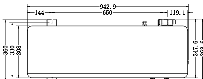
Värmepump 1402, 1403 och 1404
