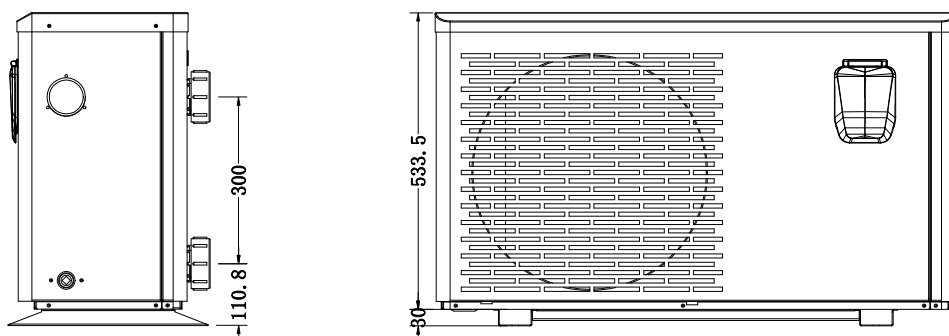
Värmepump 1401
