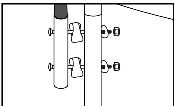
3. Spænd bolte som vist på billedet, så bundrør kommer til at sidde fast på ben.
